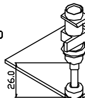
AQNA-3178 PICK-UP NOZZLE \phi 7.0 (OD= \phi 7.0 ) FUJI , IP3
