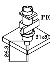
AQNA-3332 PICK-UP NOZZLE \phi 6.5 (OD= \phi 6.5 ) FUJI , IP3
