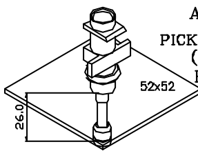
AQNA-3209 PICK-UP NOZZLE \phi 20.0 (OD= \phi 20.0 ) FUJI , IP3
